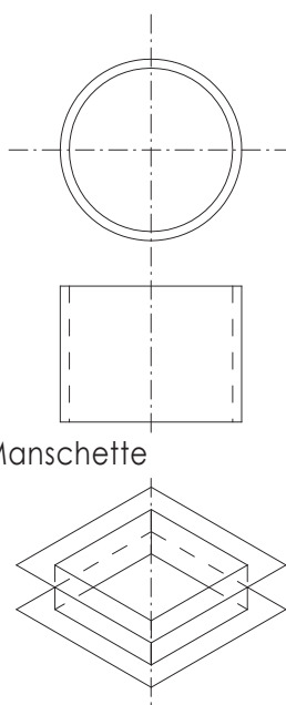
Kompensator
