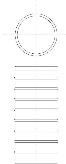
einfacher Verladeschlauch mit Drahringen, innen glatt
