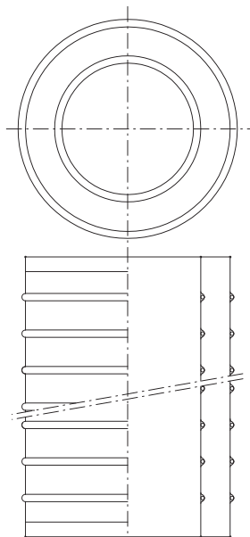
Außen- und Innenschlauch ohne Verbindung
