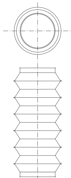
Verladeschlauch mit Ringen und umgelegten Spiralfedern
