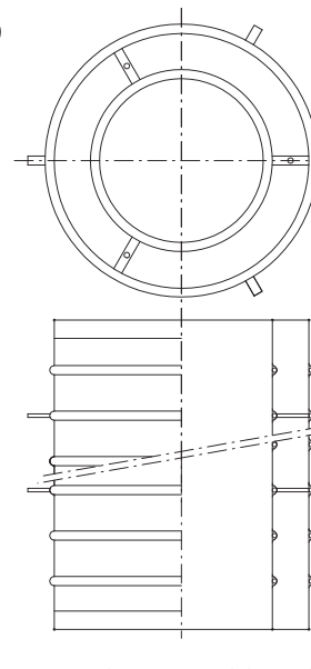
Außen- und Innenschlauch mitein- ander verbunden Außenschlauch mit Seilführungsstegen
