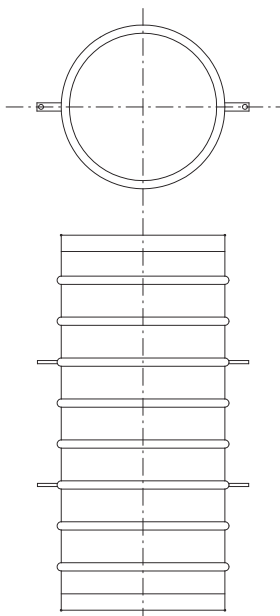
Verladeschlauch mit Ringen und Seil- führungsstegen gegenüberliegend
