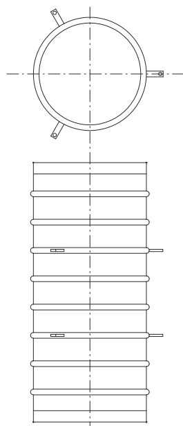
Verladeschlauch mit Ringen und Seil- führungsstegen 120° versetzt
